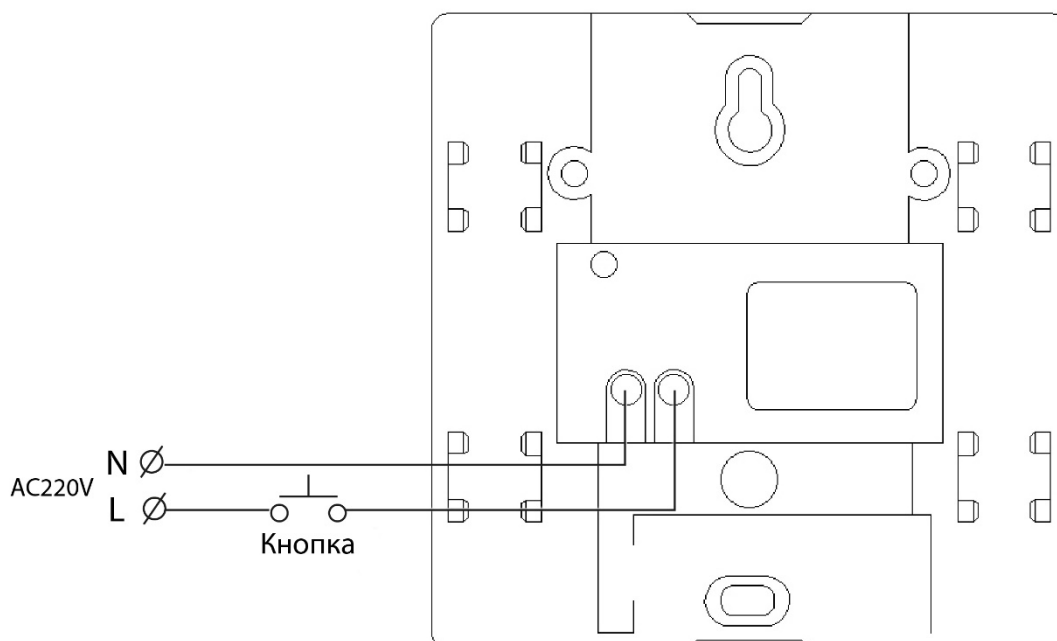
Схема подключения
